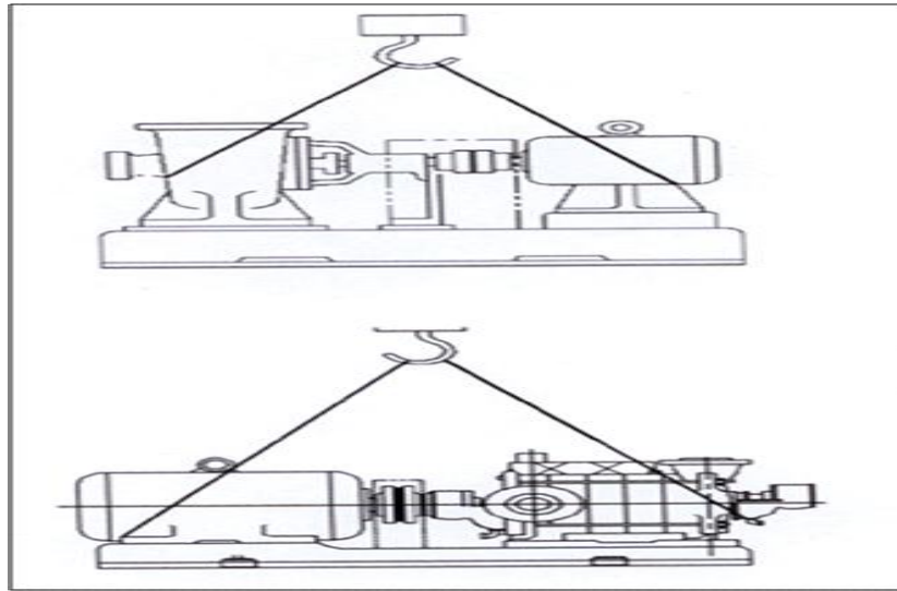
펌프의 운반방법
